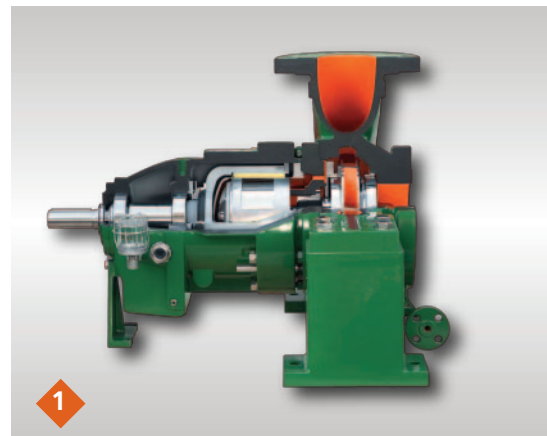
Centrifugaalpomp type PRM volgens API 685 Met magneetkoppeling.
