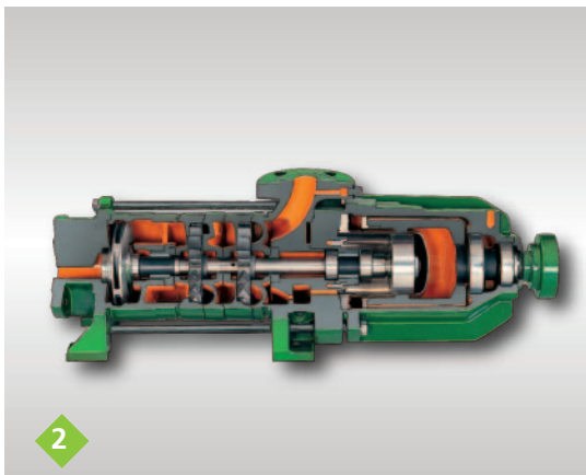
Zijdekanaalpomp type SC / SCM Met mechanische asafdichting of magneetkoppeling.
