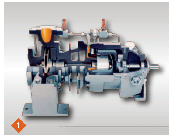
Centrifugaalpomp type NMWR / PRMW voor thermische olie Met magneetkoppeling voor temperaturen tot 450°C.
