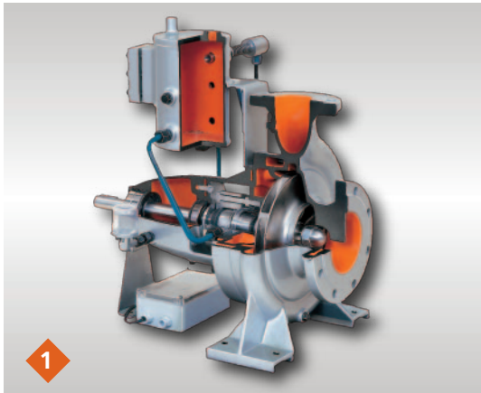
Centrifugaalpomp type NCL (volgens EN- en ISO-normen) Met mechanische asafdichting.
