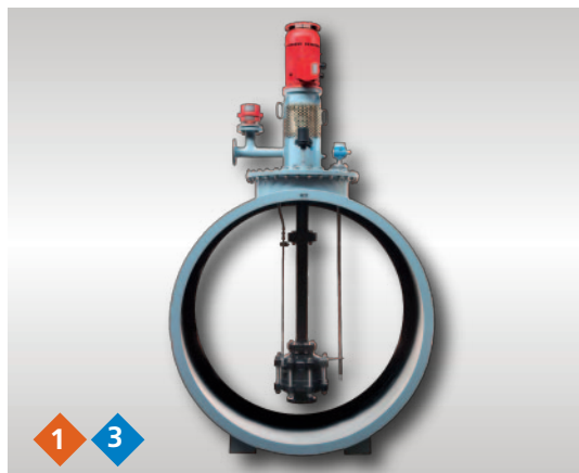
Verticale één- of meertraps staartpomp type NCT / HZV / NMT Met mechanische asafdichting of magneetkoppeling. Geschikt voor ATEX Zone 0.
