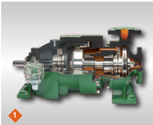
Centrifugaalpomp type NMR / NML / NMB volgens EN- en ISO-normen Met magneetkoppeling.
