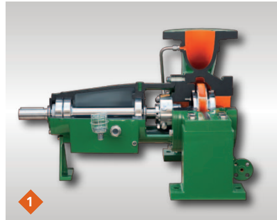
Centrifugaalpomp type NCR volgens API 610 Met mechanische asafdichting.
